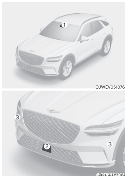
[1] : Caméra frontale, [2] : Radar avant [3] : radar d'angle avant (si équipé)
