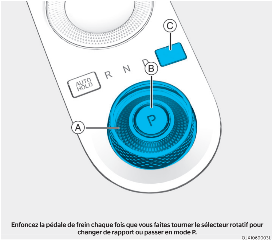
[A] : Sélecteur rotatif (sélecteur rotatif de rapport), [B] : Bouton P [C] : Cache P-release
