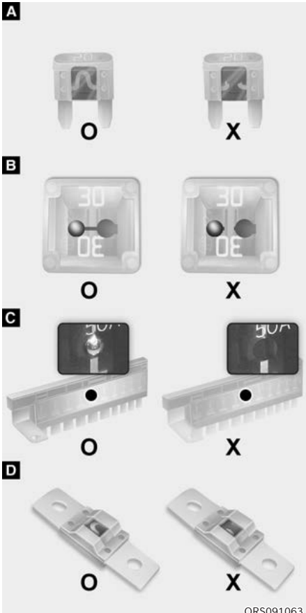
[A]: Flachsicherung, [B]: Patronensicherung, [C]: Mehrfachversicherung, [D]: Midi-Sicherung O: Normal, X: Durchgebrannt
