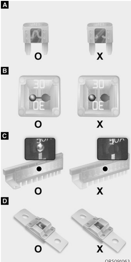
[A]: Flachsicherung, [B]: Patronensicherung, [C]: Mehrfachsicherungen, [D]: Midi-Sicherung O: Normal, X: Durchgebrannt
